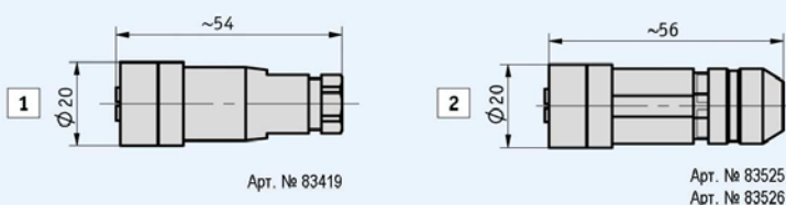
Ответные части разъемов прямые
