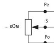
Потенциометрические выходы P01, P05, P10
