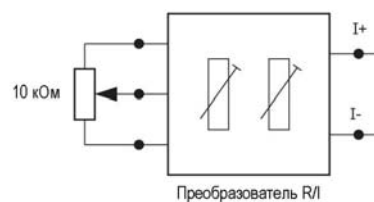
Измерительный преобразователь MWU
