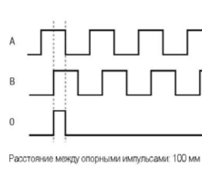
Инкрементальный датчик
