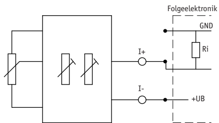
Abb. 3: Anschluss Bürde gegen +UB
